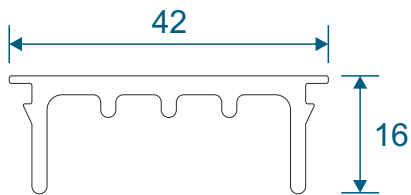
IMP301 - Infill Strip
