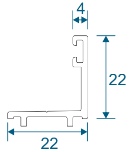
VG12 - External Door Bead
